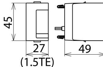
Maßbild DG MOD E DC 550
