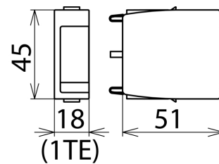
Maßbild DG MOD CI 275
