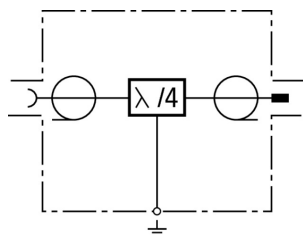
Prinzipialschaltbild DGA L4 7 16 MFA
