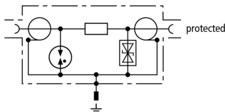
Prinzipschaltbild DGA BNC VCD
