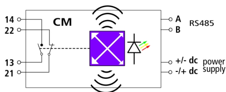
Prinzipschaltbild DRC MCM XT
