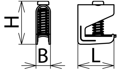
Maßbild SAK
