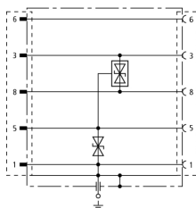
Prinzipialschaltbild FS 9E PB 6
