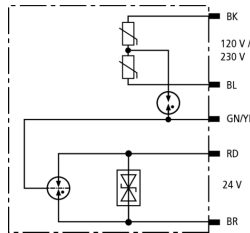
Prinzipialschaltbild DPI CD EXD 230 24 M
