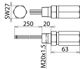
Maßbild DPI CD EXD 230 24 M
