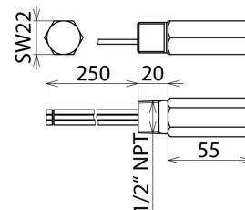
Maßbild DPI CD EXD 24 N
