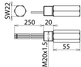
Maßbild DPI CD EXD 24 M
