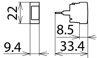
Maßbild DRL HD 5
