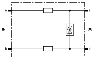
Prinzipialschaltbild DRL HD 5
