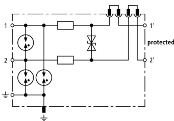
Principalschaltbild DCO SD2 MD EX 24
