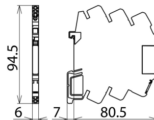
Maßbild DCO SD2 E 24
