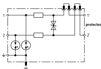
Prinzipschaltbild DCO SD2 MD 12
