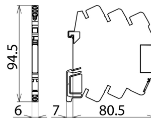
Maßbild DCO SD2 ME 12
