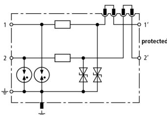
Prinzipialschaltbild DCO SD2 ME 12
