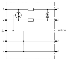
Prinzip Schaltbild BSP M2 BD 60
