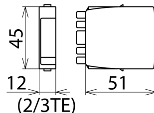
Maßbild BSP M2 BD 60
