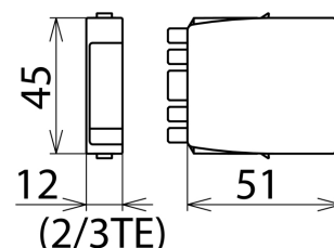
Maßbild BSP M2 BD 48
