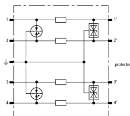
Prinzipschaltbild BSP M4 BE HF 5
