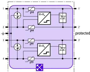
Principalschaltbild BXTU ML4 BD 0-180
