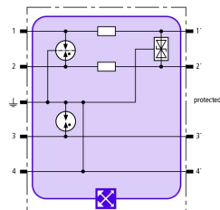
Principalschaltbild BXT ML2 BE HFS 5
