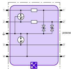
Principalschaltbild BXT ML2 BE S 36
