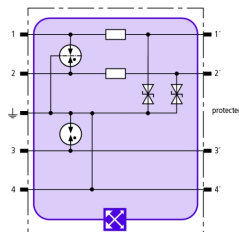
Prinzipschaltbild BXT ML2 BE S 24
