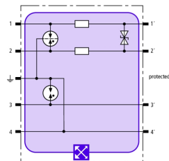
Principalschaltbild BXT ML2 BD S 48
