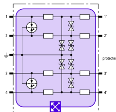
Principalschaltbild BXT ML4 BE C 24
