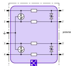
Prinzipschaltbild BXT ML4 BD 180
