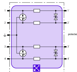
Prinzipschaltbild BXT ML4 BD 48
