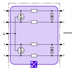
Prinzip Schaltbild BXT ML4 BD 5
