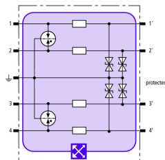
Prinzipschaltbild BXT ML4 BE 48
