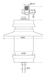
Maßbild DTR 3.6 10 3
