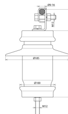
Maßbild DTR 1.2 10 3
