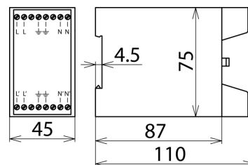
Maßbild NF 10
