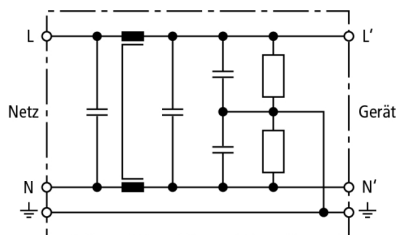
Prinzipialschaltbild NF 10
