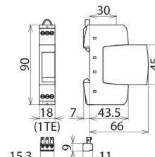
Maßbild DR M 2P 75 FM
