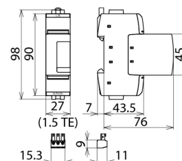
Maßbild DG SE H LI 440 FM
