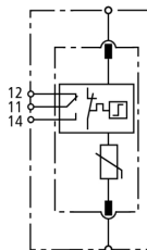
Principalschaltbild DG S 385 FM
