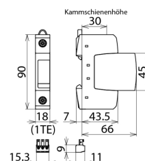
Maßbild DG S CI 275 FM
