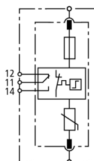
Prinzipialschaltbild DG S CI 275 FM
