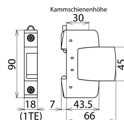
Maßbild DG S CI 275
