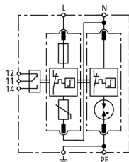
Prinzip Schaltbild DG M TT 2P CI 275 FM
