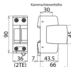
Maßbild DG M TT 2P CI 275
