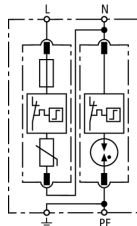
Prinzipialschaltbild DG M TT 2P CI 275
