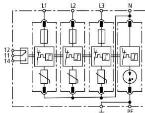
Prinzipschaltbild DG M TT CI 275 FM
