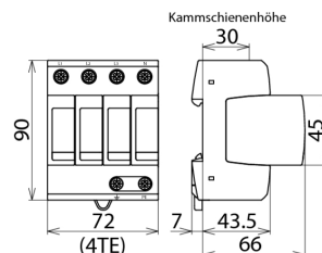
Maßbild DG M TT CI 275
