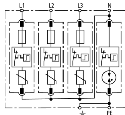
Prinzipschaltbild DG M TT CI 275
