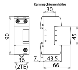
Maßbild DB M 1 320
