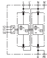
Principalschaltbild DV M TT 2P 255 FM
