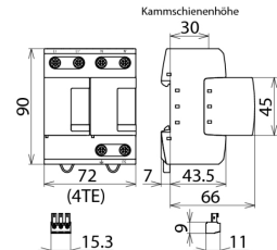
Maßbild DV M TT 2P 255 FM
