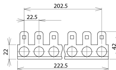
Maßbild MB2 10 LSA
